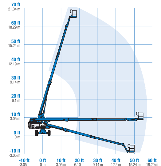
Biểu đồ hoạt động cần Boom S™-65
