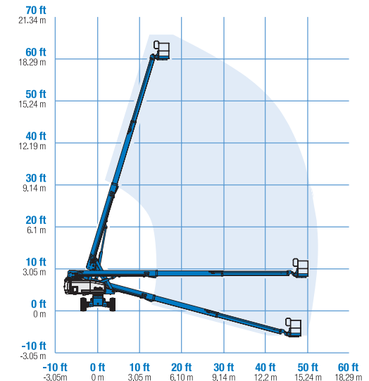
Biểu đồ hoạt động cần Boom S™-60
