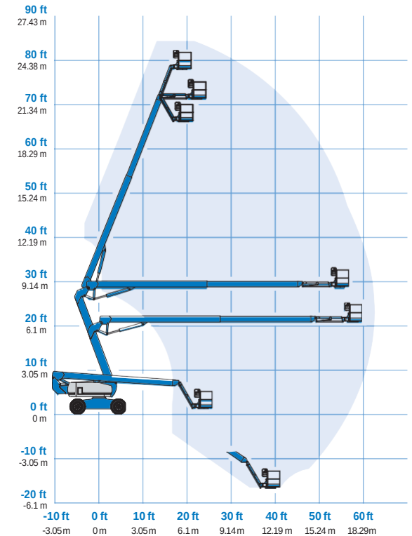
Biểu đồ hoạt động cần Boom Z-80/60
